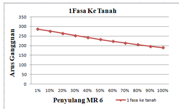
Gambar 16. Kurva arus hubung singkat 1fasa ke tanah (MR 6)
