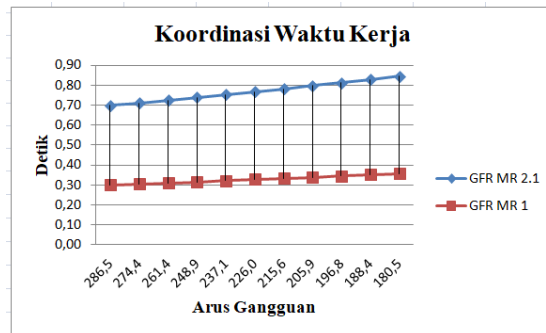
Gambar 21. Kurva waktu kerja relai GFR MR 2.1 dan GFR MR 1
