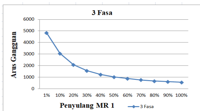
Gambar 9. Kurva arus hubung singkat 3 fasa (MR 1)
