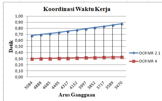
Gambar 19. Kurva waktu kerja relai OCR MR 2.1 dan OCR MR 4
