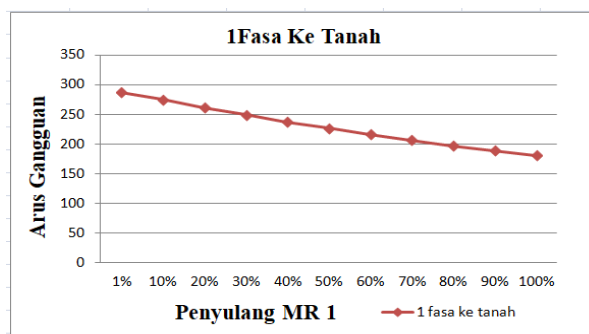
Gambar 10. Kurva arus hubung singkat 1fasa ke tanah (MR 1)
