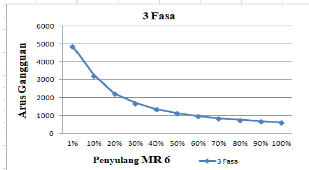
Gambar 15. Kurva arus hubung singkat 3 fasa (MR 6)
