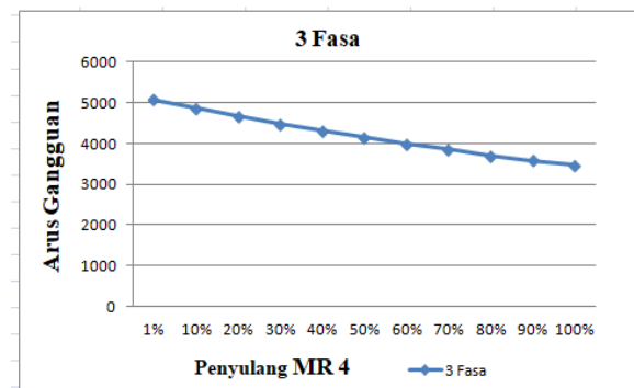
Gambar 13. Kurva arus hubung singkat 3 fasa (MR 4)
