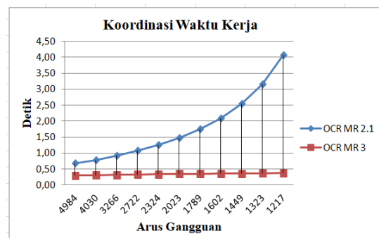
Gambar 18. Kurva waktu kerja relai OCR MR 2.1 dan OCR MR 3
