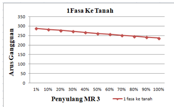
Gambar 12. Kurva arus hubung singkat 1fasa ke tanah (MR 3)
