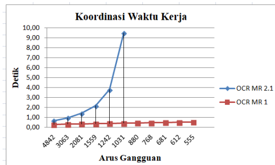
Gambar 17. Kurva waktu kerja relai OCR MR 2.1 dan OCR MR 1
