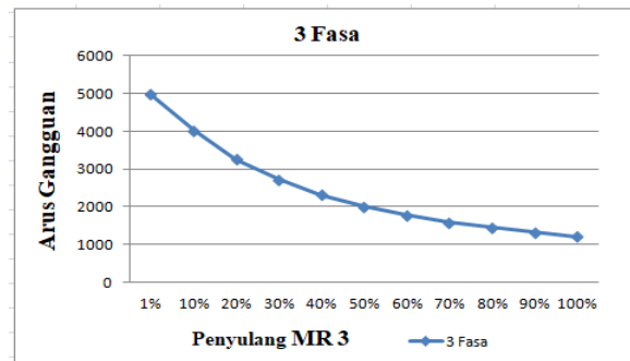
Gambar 11. Kurva arus hubung singkat 3 fasa (MR 3)
