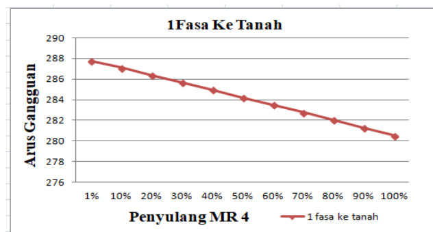
Gambar 14. Kurva arus hubung singkat 1fasa ke tanah (MR 4)
