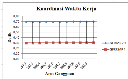
Gambar 23. Kurva waktu kerja relai GFR MR 2.1 dan GFR MR 4
