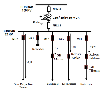
Gambar 3. Singeline Gardu Induk Marisa 20 kV
