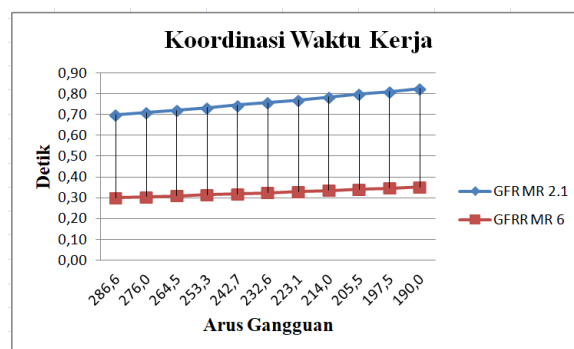
Gambar 24. Kurva waktu kerja relai GFR MR 2.1 dan GFR MR 6
