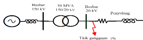
Gambar 4. Diagram satu garis untuk penyulang titik gangguan 1%
