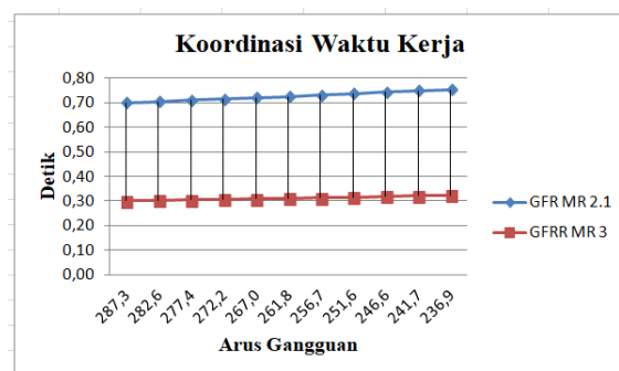
Gambar 22. Kurva waktu kerja relai GFR MR 2.1 dan GFR MR 3
